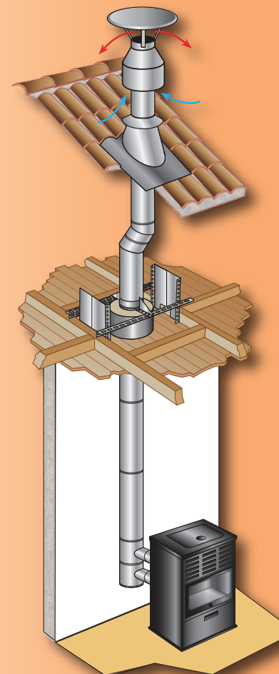
TP.5 CONDUCTO CONCÉNTRICO CONCENTRIC PIPING CONDUIT CONCÉNTRIQUE
