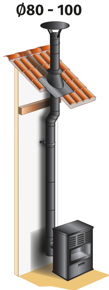
TP.2 SIMPLE PARED PINTADO NEGRO MATE SINGLE WALL, MATT BLACK SIMPLE PAROI NOIR MAT
