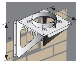
Escuadra con soporte mural Square with wall support Équerre avec support mural
