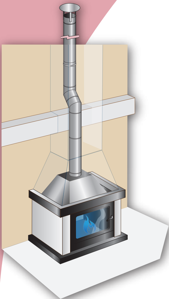
F.1 FUMISTERÍA INOXIDABLE STAINLESS STEEL CONNECTING FLUE PIPE FUMISTERIE INOXYDABLE
