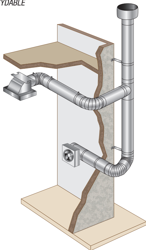
F.2 FUMISTERÍA GALVANIZADA GALVANIZED CONNECTING FLUE PIPE FUMISTERIE GALVANISÉE
