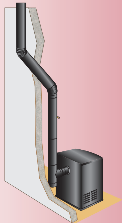
F.3 FUMISTERÍA VITRIFICADA VITREOUS ENAMEL CONNECTING FLUE PIPE FUMISTERIE ÉMAILLÉE (mate | matt | mat )
