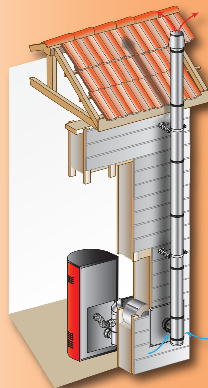
TP.4 DOBLE PARED DOUBLE WALL DOUBLE PAROI
