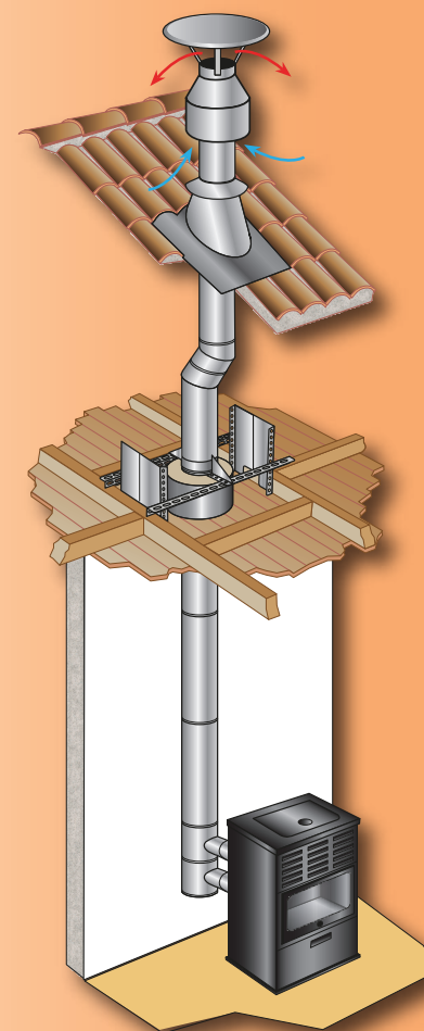
TP.5 CONDUCTO CONCÉNTRICO CONCENTRIC PIPING CONDUIT CONCENTRIQUE
