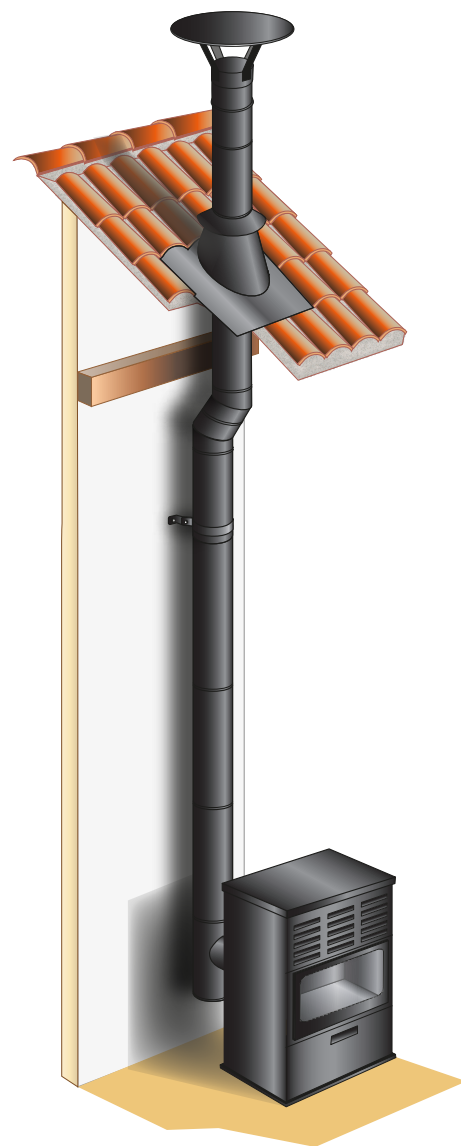
TP.2 SIMPLE PARED PINTADO NEGRO MATE SINGLE WALL, MATT BLACK SIMPLE PAROI NOIR MAT
