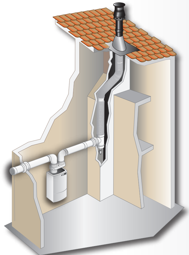
CONDUCTO FLEXIBLE BIFLUJO SIMPLE SINGLE BIFLOW FLEXIBLE DUCT CONDUIT FLEXIBLE BIFLUX SIMPLE
